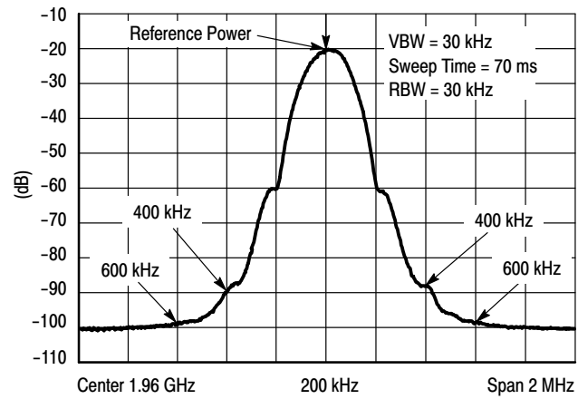
Figure 11. EDGE Spectrum
