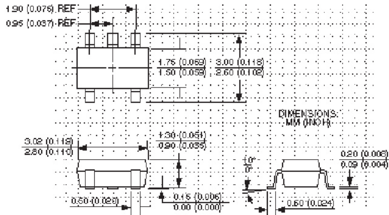
SOT-23-5 (M5)
