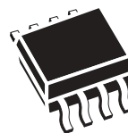
SO8 (MN) 150 mil width
