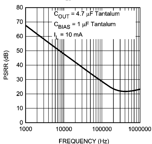
V_{IN} PSRR
