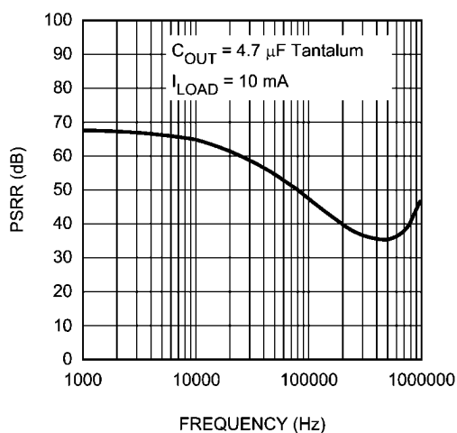
V_{BIAS} PSRR
