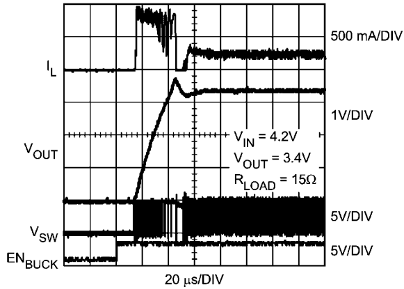
PWM Startup ( V_{CON} = 1.13\text{V} )
