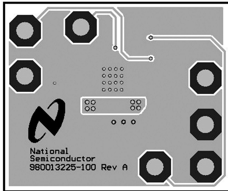
Bottom Layer
