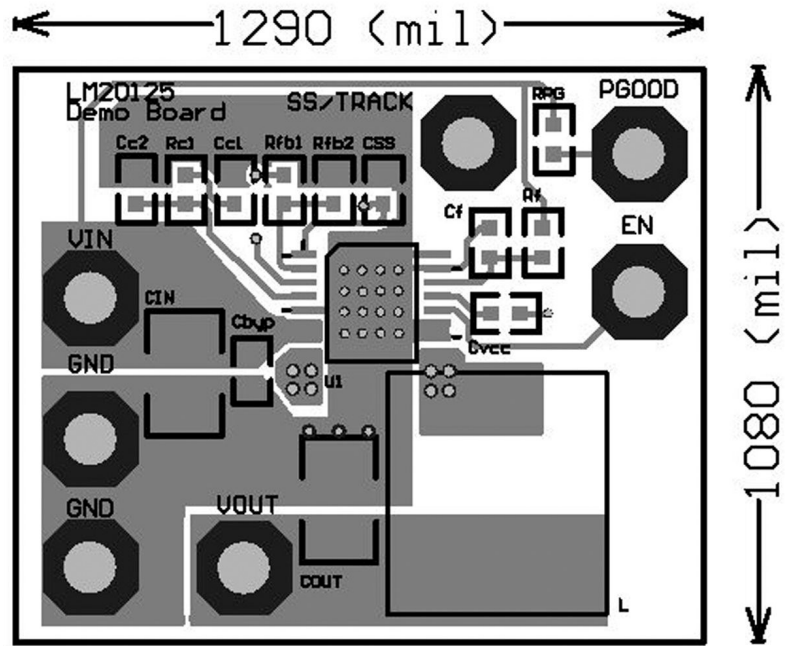
Top Layer
