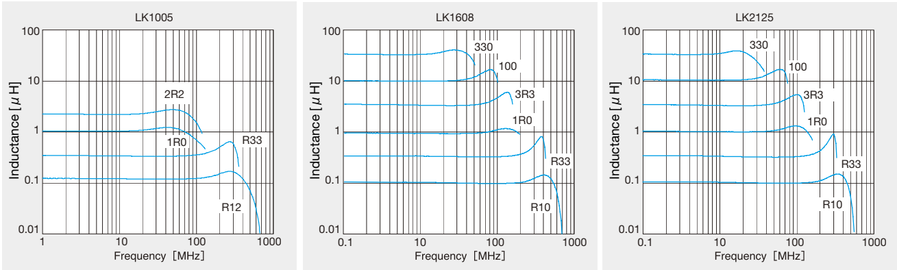
インダクタンス周波数特性例 Inductance-vs-Frequency characteristics (Measured by HP4294A or HP4291A)
