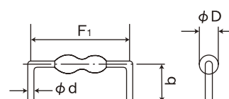
KR/KH/KB形状
