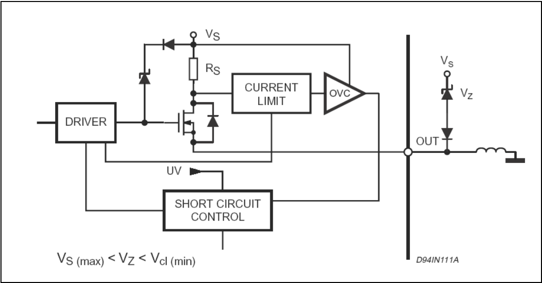
Figure 7. External demagnetisation circuit (versus V_S )
