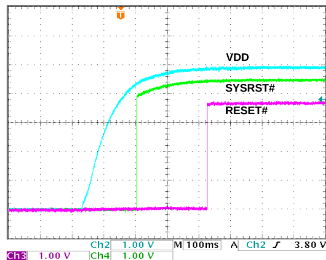
FIGURE 16. SYSRST# and RESET# vs VDD (EN = VDD, 4 UVLO > UVLO Vth)
