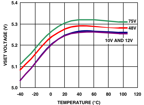
FIGURE 8. VSET VOLTAGE
