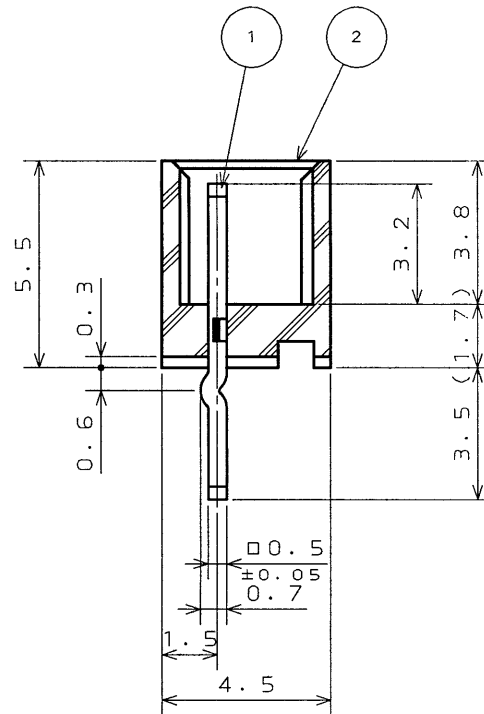
断面 A-A
