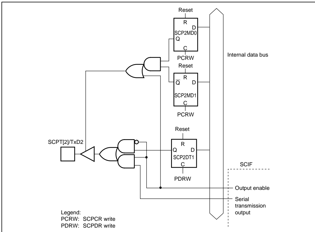
Figure 16.3 SCPT[2]/TxD2 Pin
