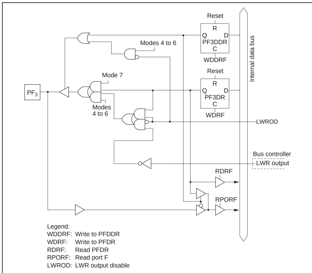
Figure C.15 (d) Port F Block Diagram (Pin PF 3 )
