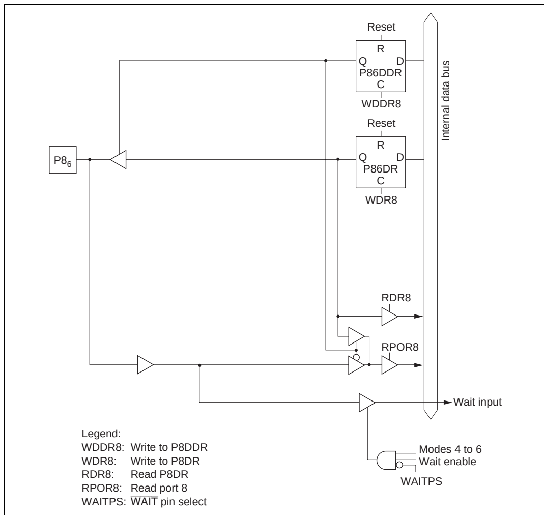
Figure C.8 (d) Port 8 Block Diagram (Pin P8 6 )
