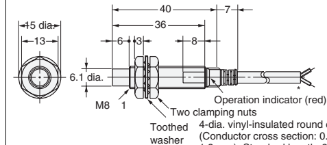
Diagram 8 E2E-X2MY□
