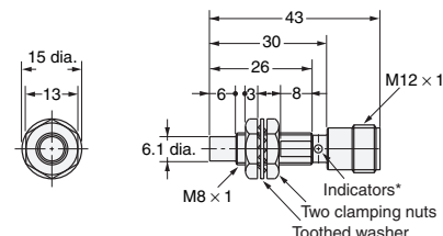
Diagram 19 E2E-X4MD□-M1(G) E2E-X2ME□-M1/E2E-X2MF□-M1
