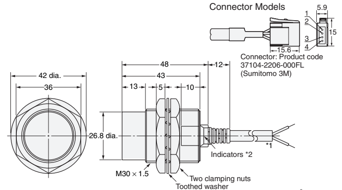
Diagram 17 E2E-X20MD□/E2E-X18ME□/F□ E2E-X18MY□
