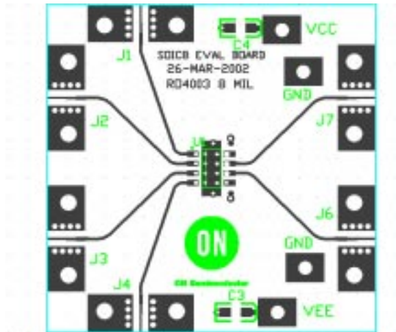
Top Layer
