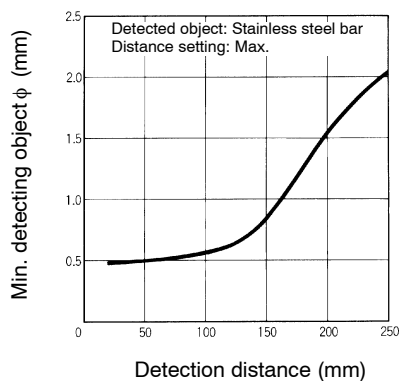
E3S-CL1
