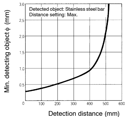
E3S-CL2
