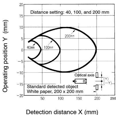
E3S-CL1
