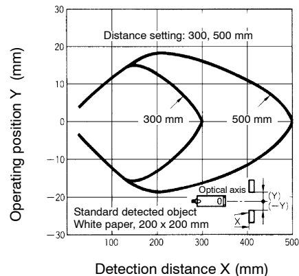
E3S-CL2
