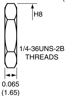
NUT
