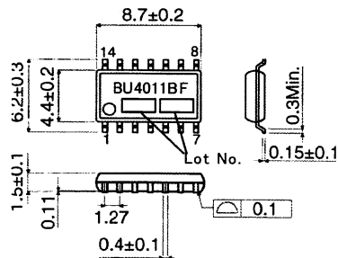
BU4011BF(SOP14)( UNIT:[mm])
