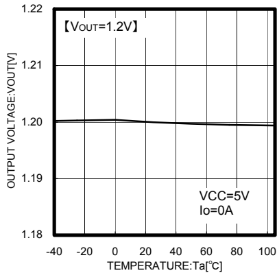
Fig.6 Ta - VOUT
