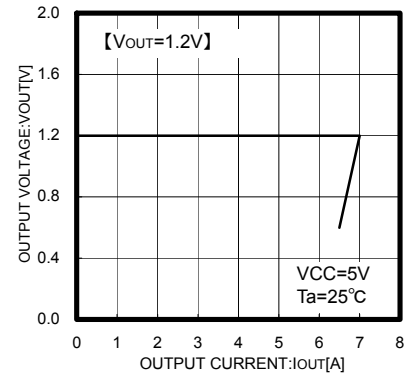
Fig.5 IOUT - VOUT
