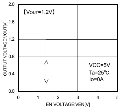
Fig.4 VEN - VOUT
