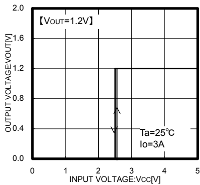
Fig.3 Vcc - VOUT
