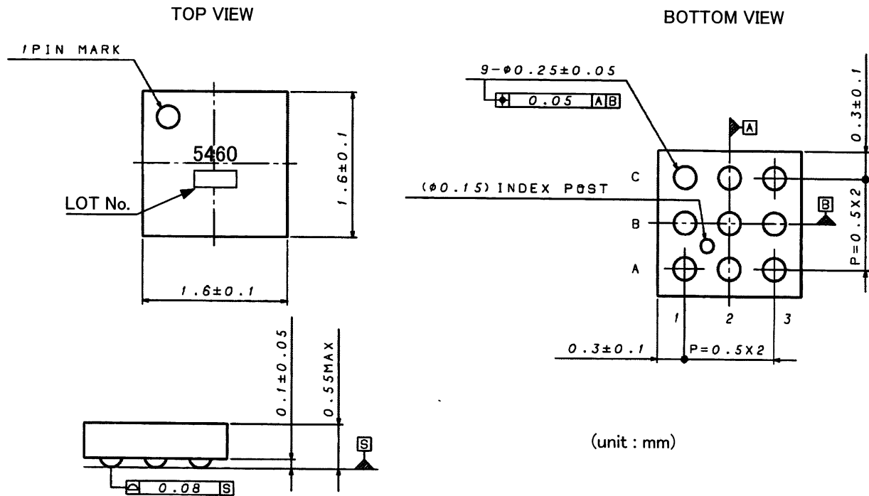
WL-CSP : VCSP50L1
