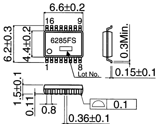
SSOP-A16 (Unit:mm)
