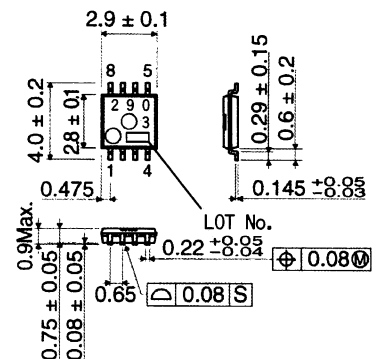
BA2903FVM (MSOP8) (Unit:[mm])
