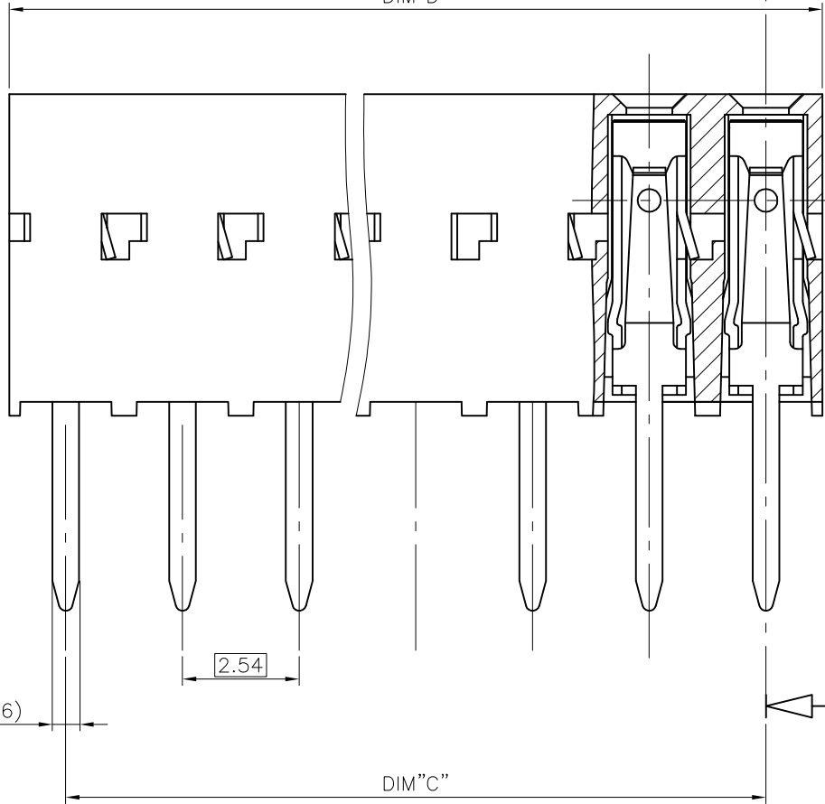
SECTION A-A
