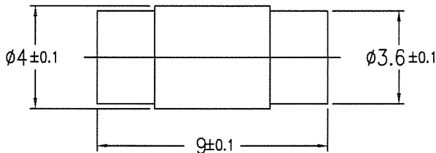
③ CRIMP SLEEVE クリンプスリーブ
