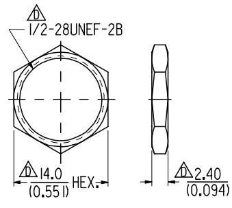
JAM NUT
