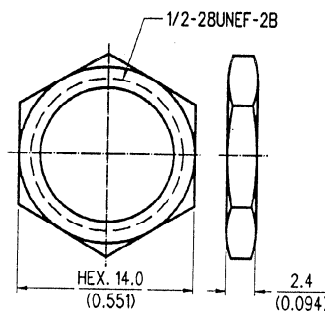
JAM NUT
