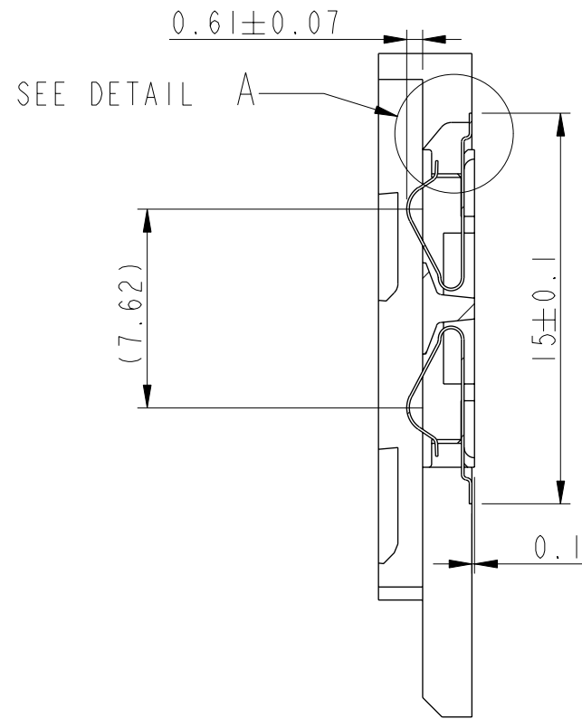
SECTION A-A
