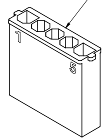
43680-*005 (NO SCALE)
