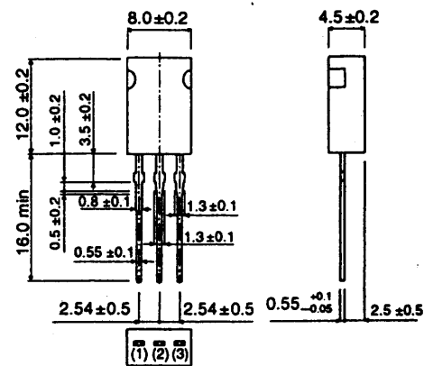
2SD2096 (HRT)
