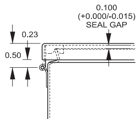
Hinge Side
