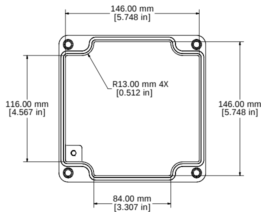
LID - INSIDE
