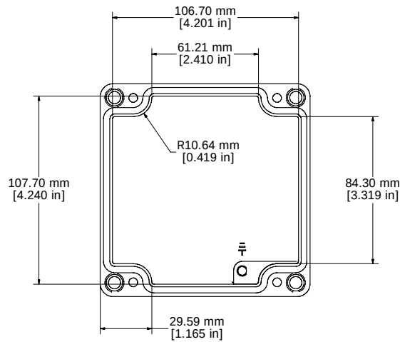
LID - INSIDE
