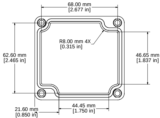
LID - INSIDE
