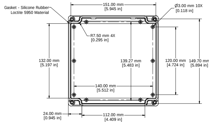
LID - INSIDE
