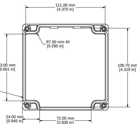
LID - INSIDE
