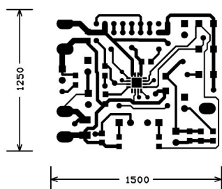
Top Gerber
