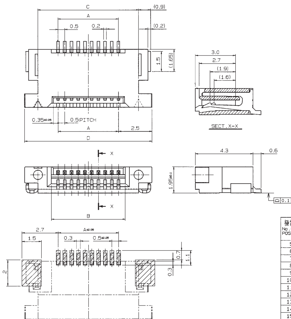
推奨基板取付け寸法 (コネクタ搭載側)
