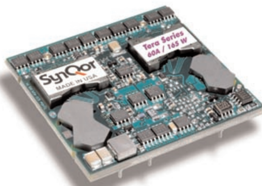
PQ48033HTA50 Module
