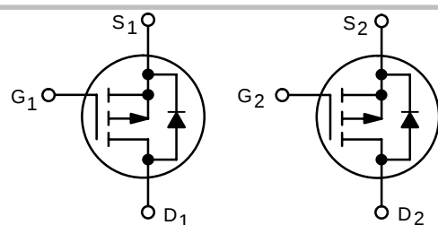
P-Channel MOSFET
