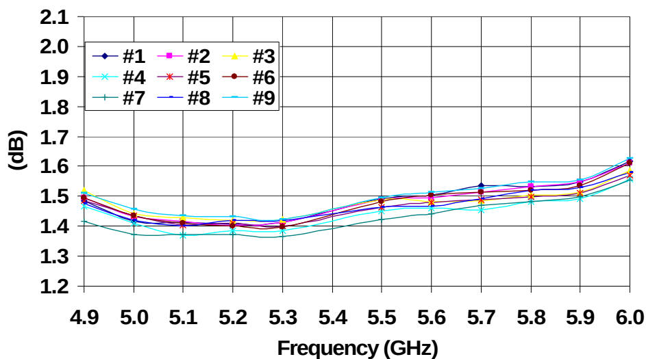
5.2 GHz LNA NF (25C)
