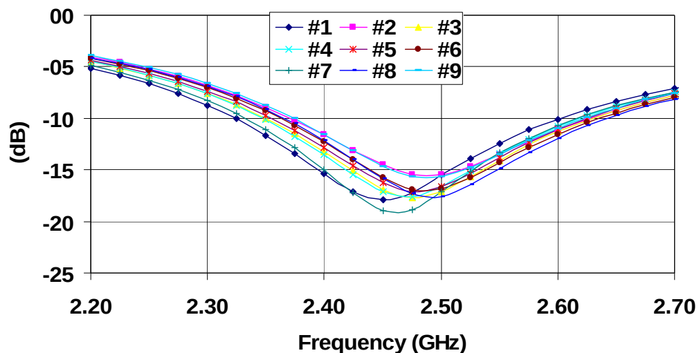
2.4 GHz LNA Output Match (25C)
