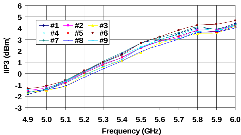
5.2 GHz LNA IIP3 (25C)
