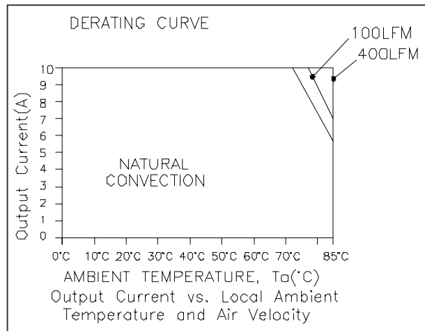
S7BC-10E2Ax, V_o=1.8\text{V}
