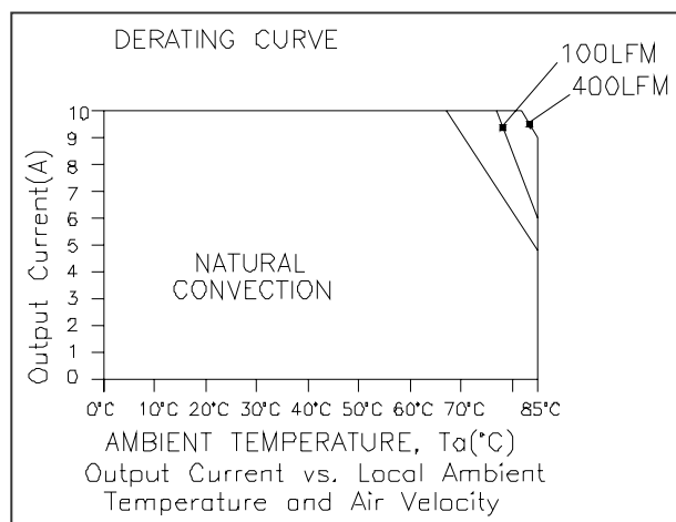
S7BC-10E2Ax, V_o=3.3\text{V}
